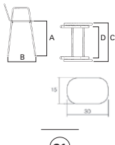
aggancio tavoletta tablet hook
